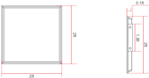
Montaje Empotrado
